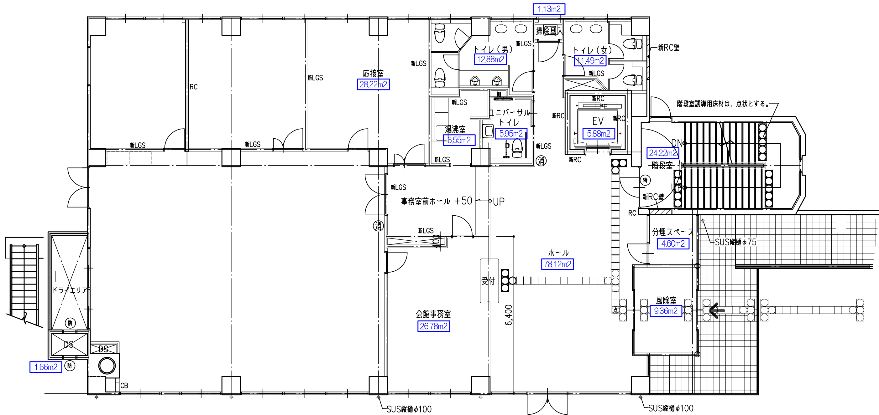
1階平面図
